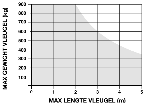
GRAFIEK 1 (mod. XLFAB5024)
